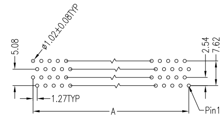
P.C.B. Layout (±0.05)
